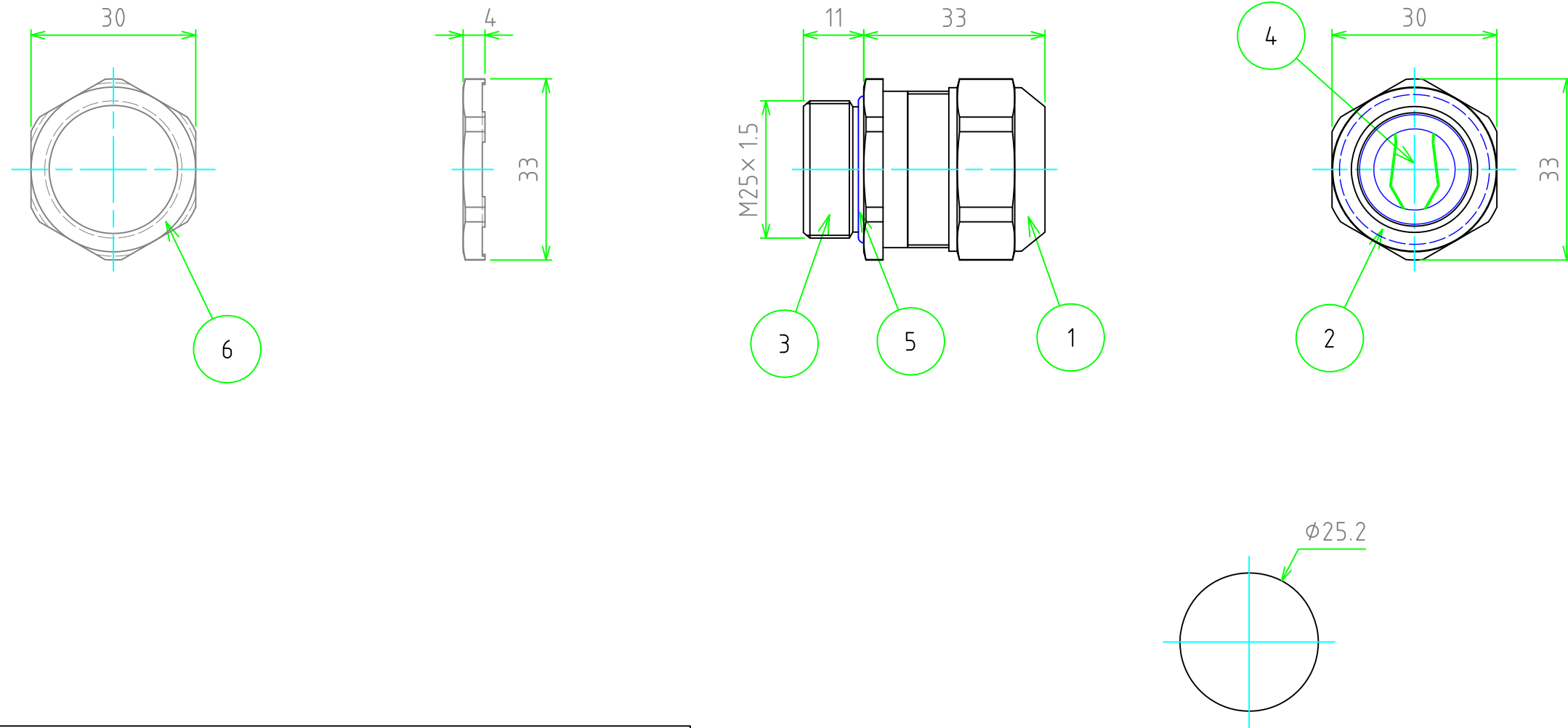
取付穴寸法 / Mounting hole dimensions
