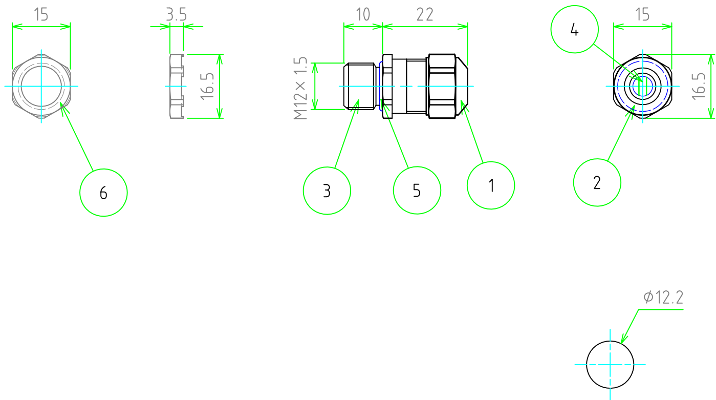
取付穴寸法 / Mounting hole dimensions
