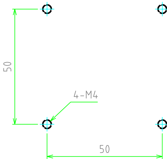
取付穴寸法
