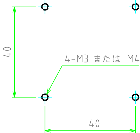
取付穴寸法
