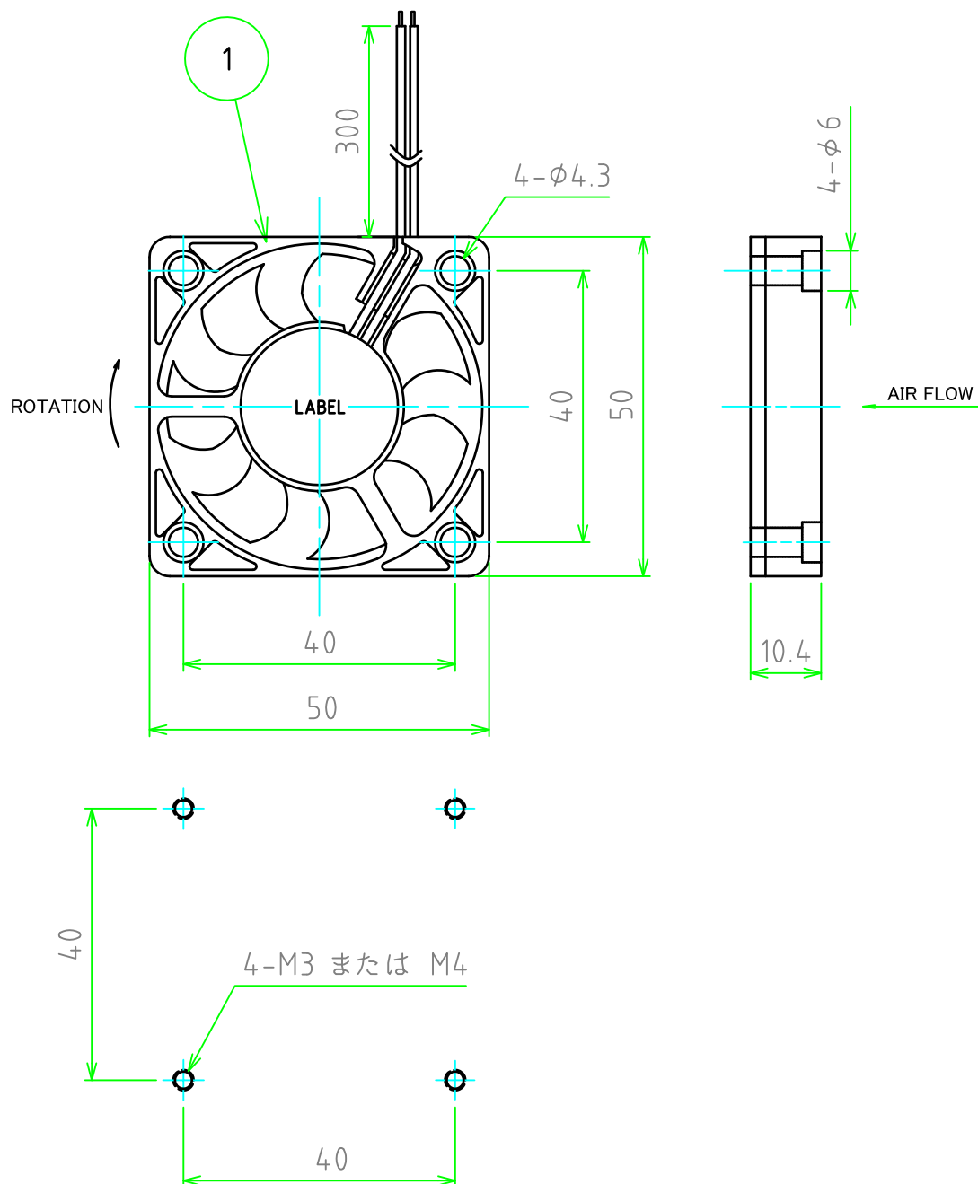
取付穴寸法
