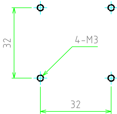
取付穴寸法
