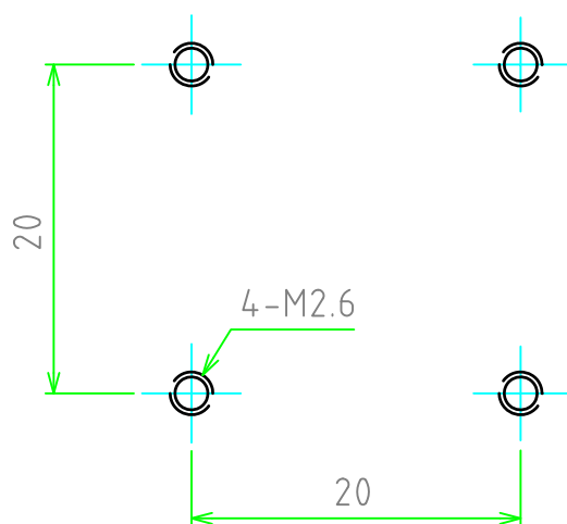
取付穴寸法
