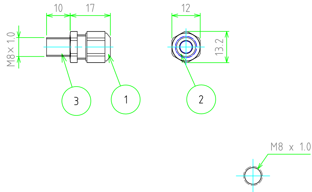
取付穴寸法 / Mounting hole dimensions
