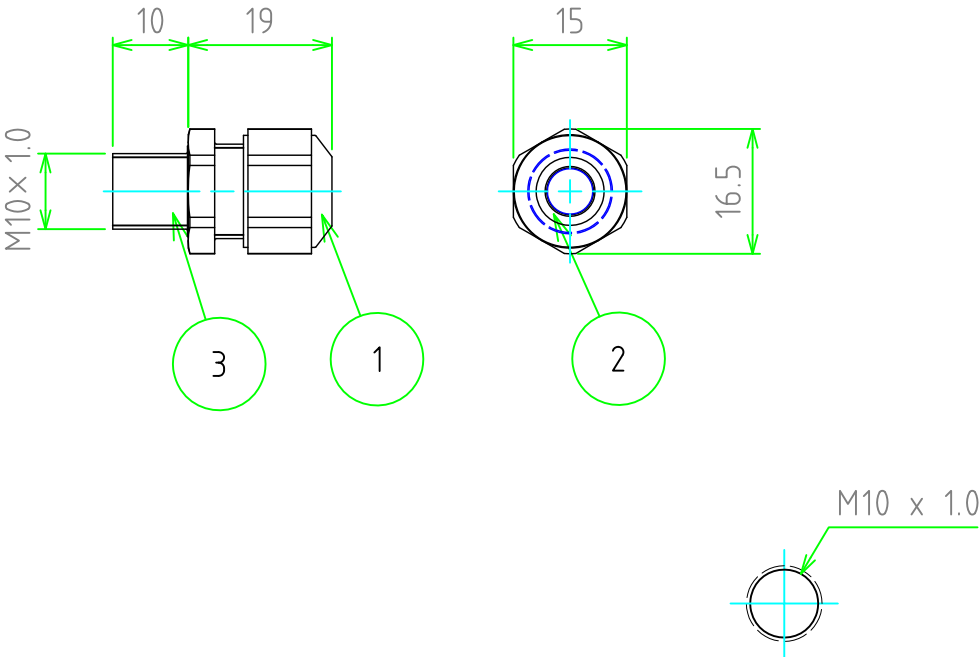
取付穴寸法 / Mounting hole dimensions
