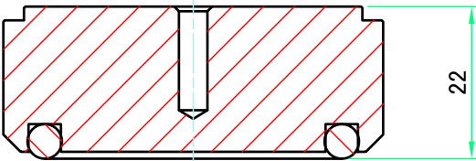
A-A (1:1)
