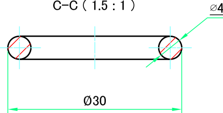
C-C ( 1.5 : 1 )
