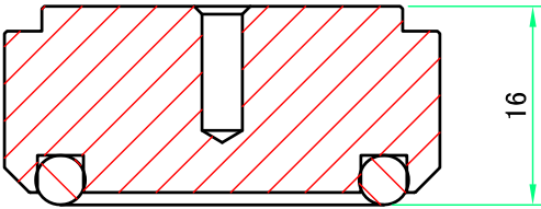
A-A ( 1.5 : 1 )
