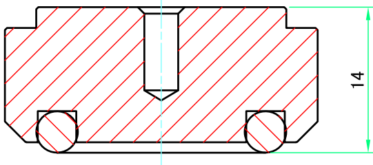
A-A ( 2 : 1 )
