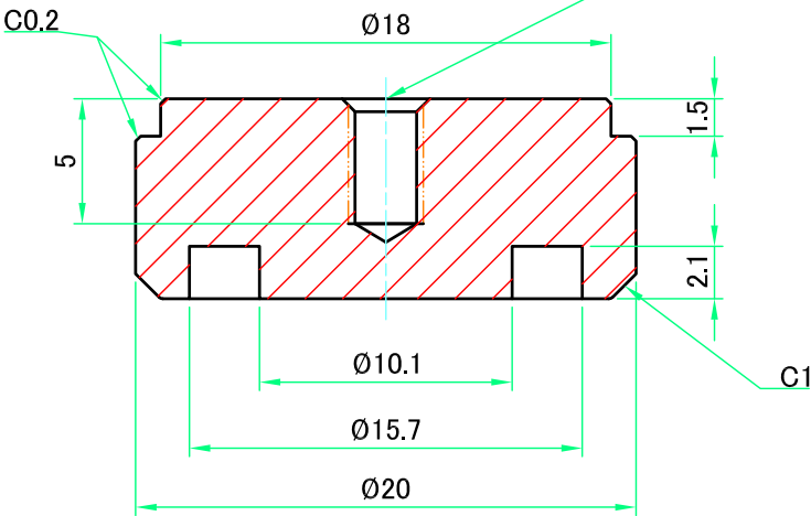
B-B ( 3 : 1 )
