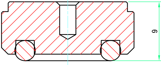
A-A ( 3 : 1 )
